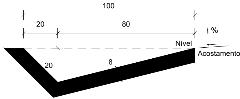
Seção transversal Escala 1 : 20
