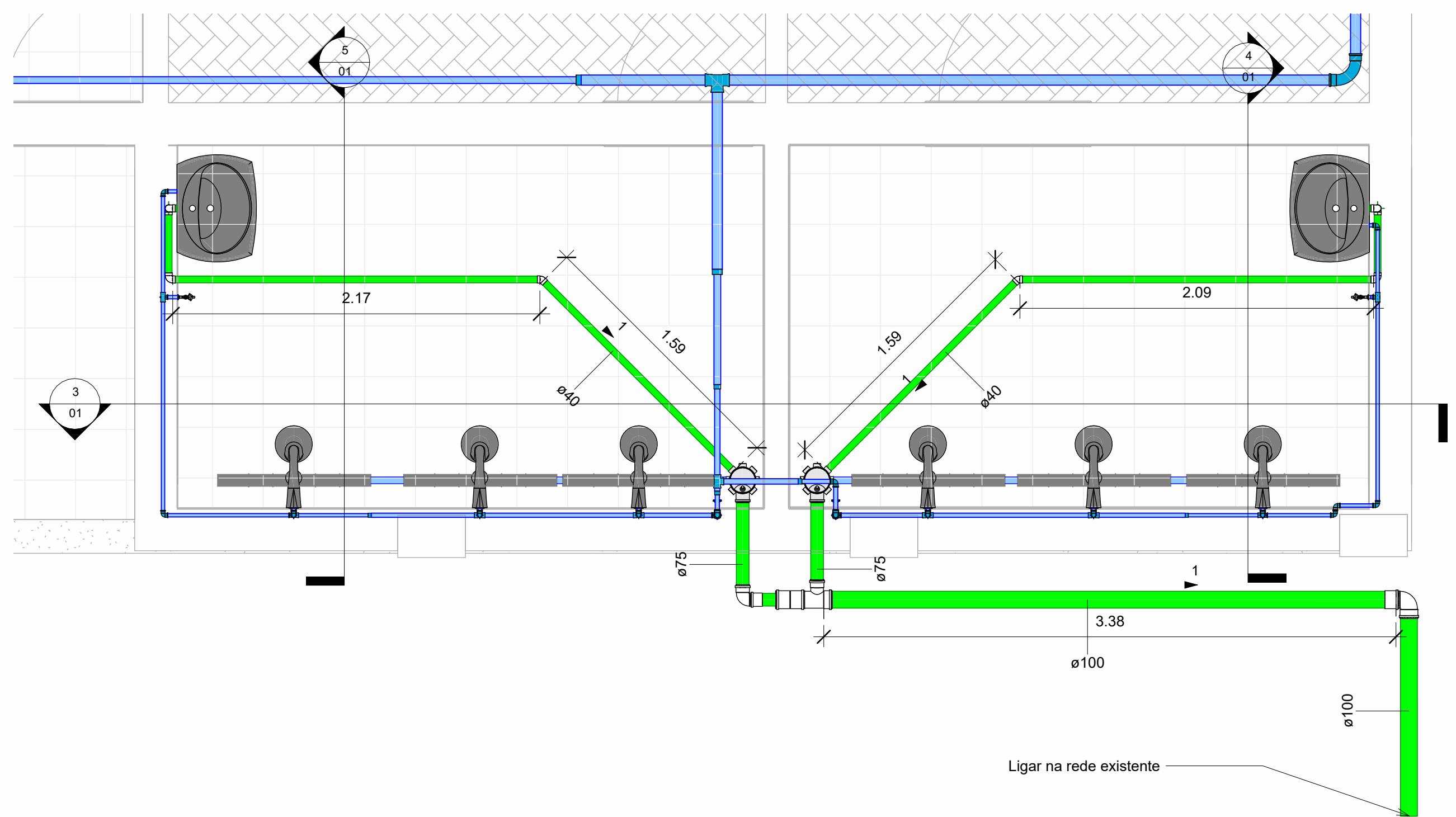
2 Planta Chuveiros 1 : 25
