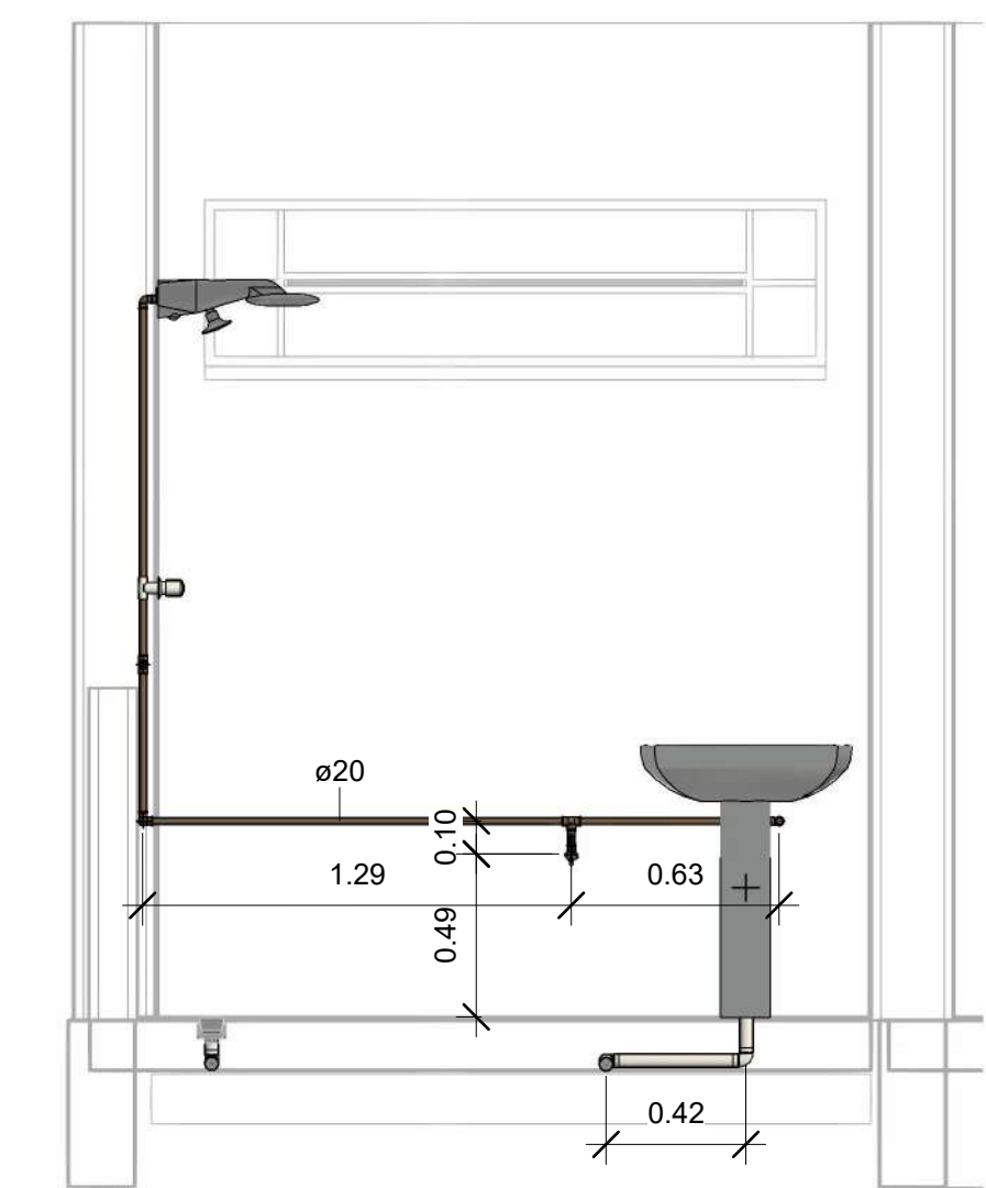
5 Corte 03 1 : 25
