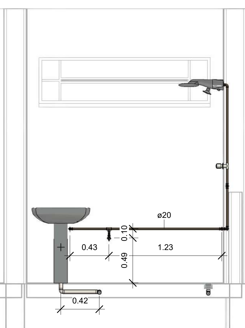
4 Corte 02 1 : 25
