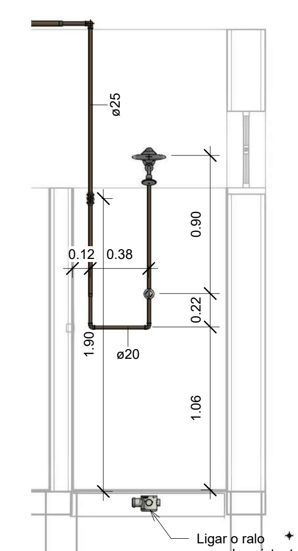
7 Corte 04 1 : 25
