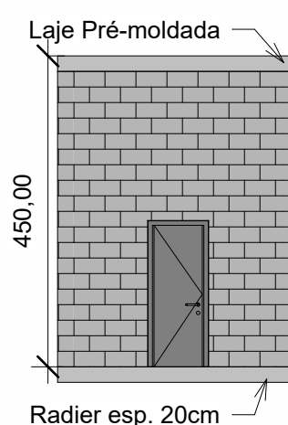
Vista 1 Res. 1 : 100
