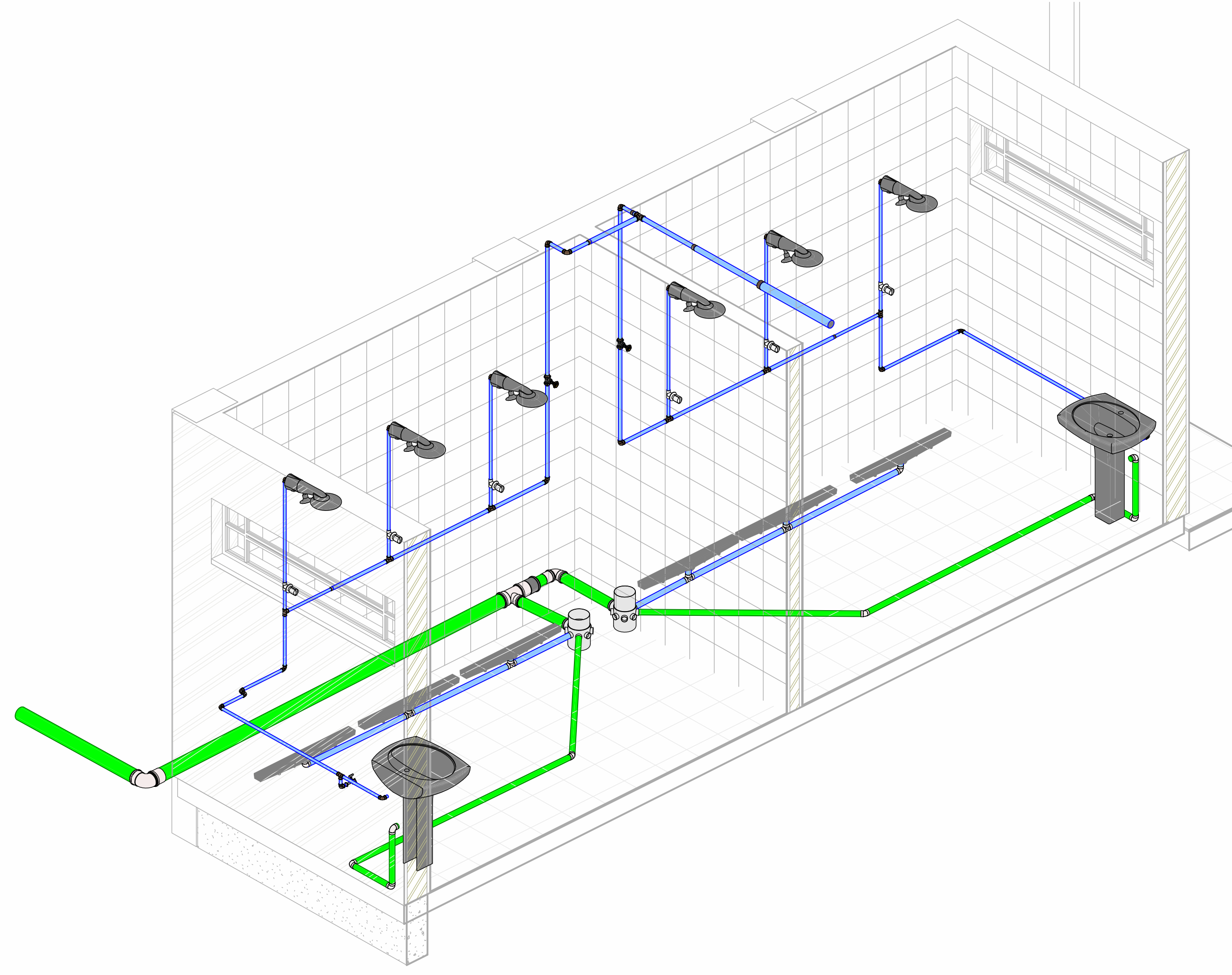
10 Chuveiros
