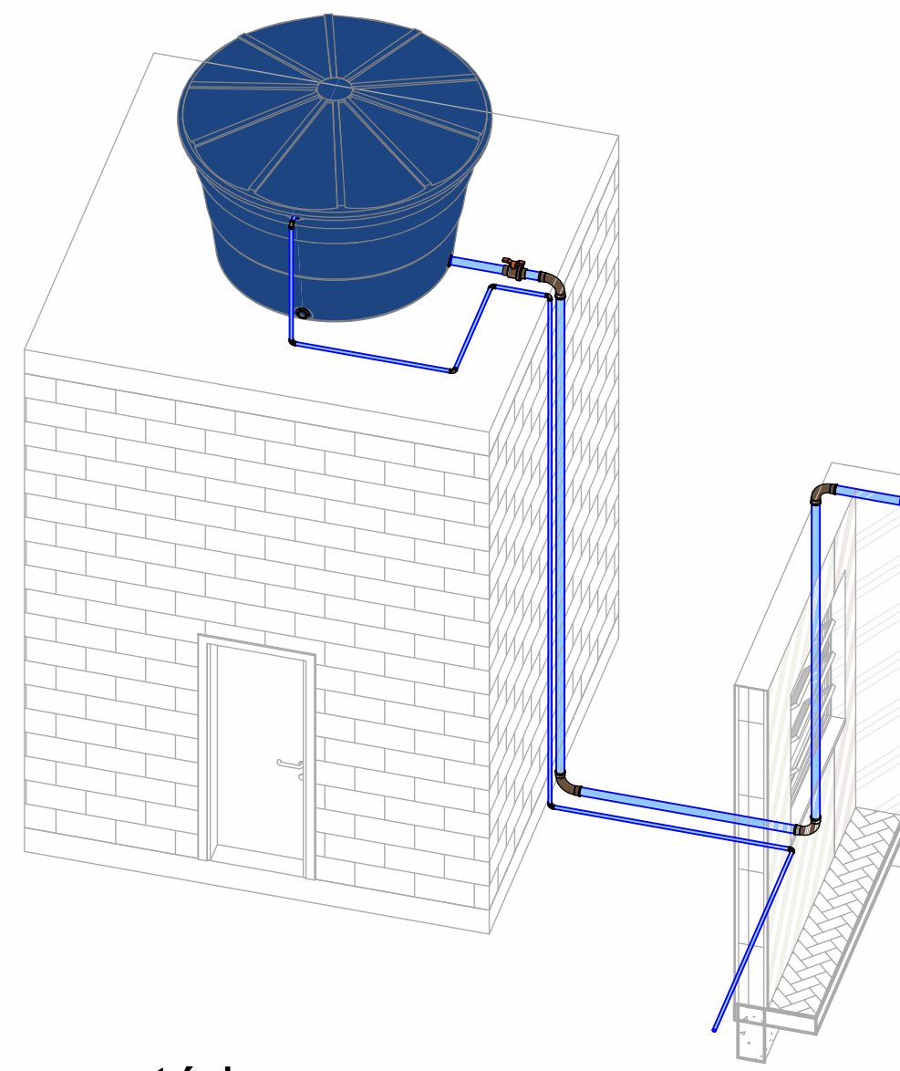
11 Reservatório
