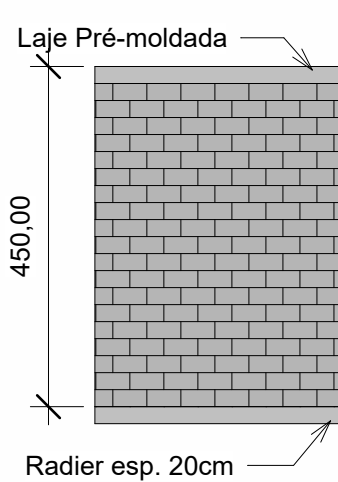
Vista 2 Res. 1 : 100
