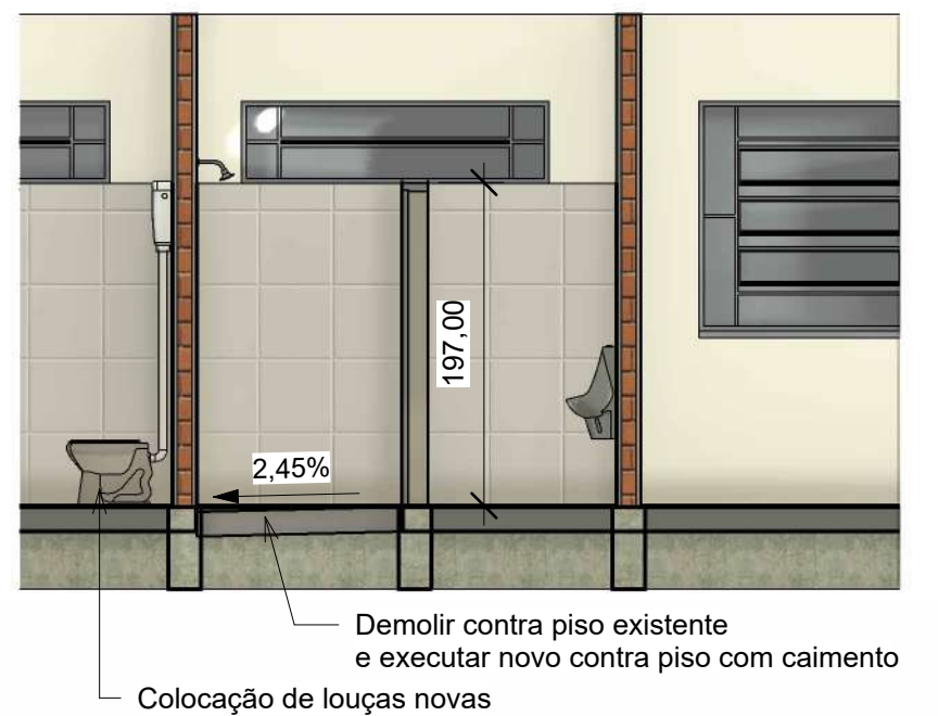
7 Corte 5 1 : 50
