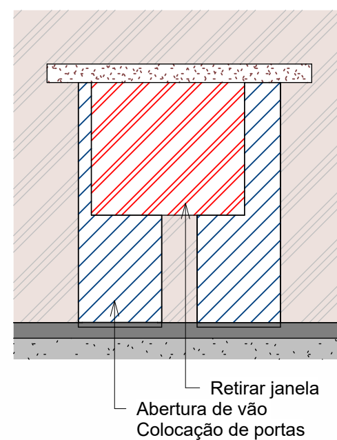
9 Corte 6 - Chamada de detalhe 1 1 : 50
