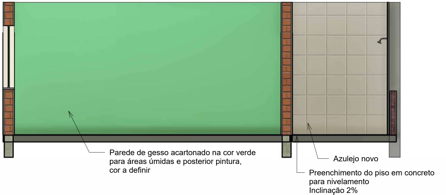
3 Corte 2 1 : 50
