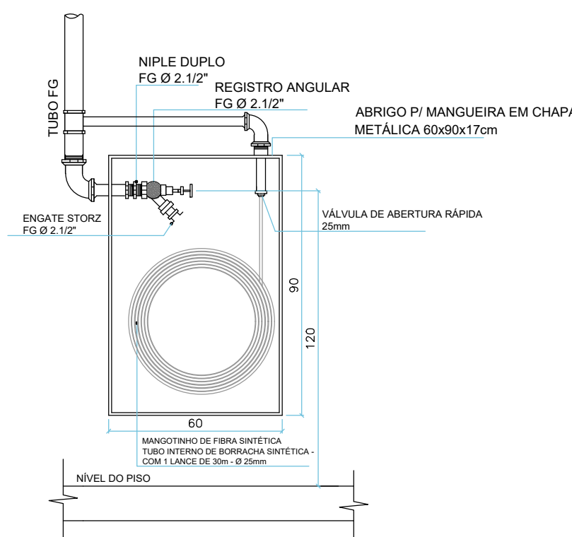
CORTE AA
