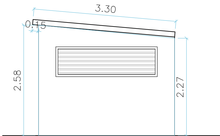
VISTA LATERAL CASA BOMBAS ESCALA: 1/50
