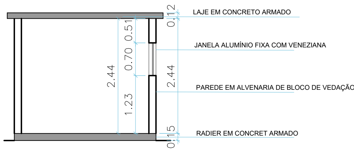
CORTE CASA BOMBAS ESCALA: 1/50
