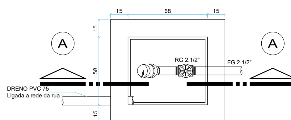
PLANTA BAIXA
