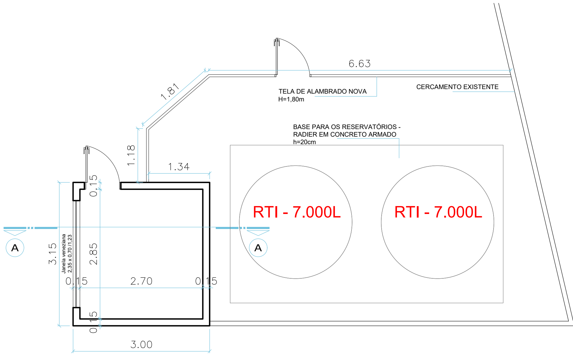
PLANTA BAIXA CASA BOMBAS ESCALA: 1/50
