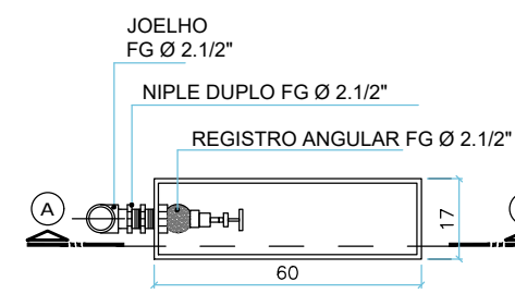
PLANTA BAIXA - HIDRANTE DUPLO
