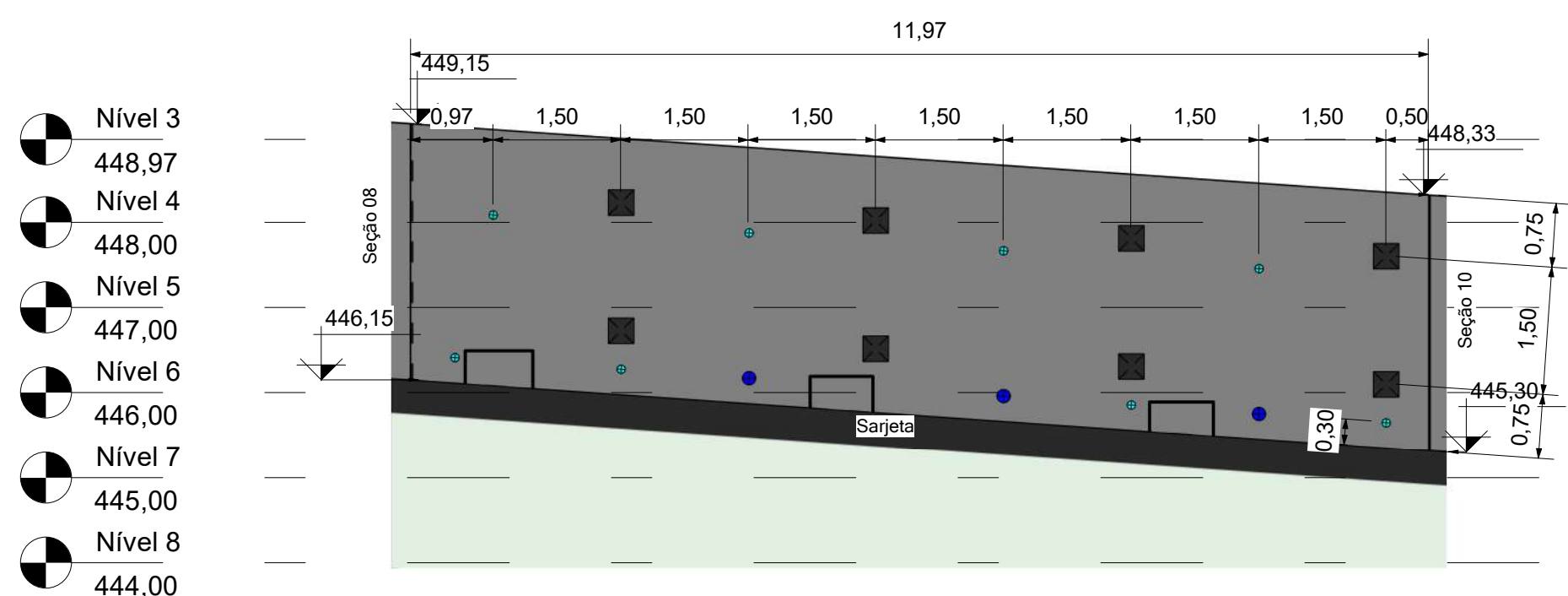
9 Seção 09 - Vista frontal 1 : 75
