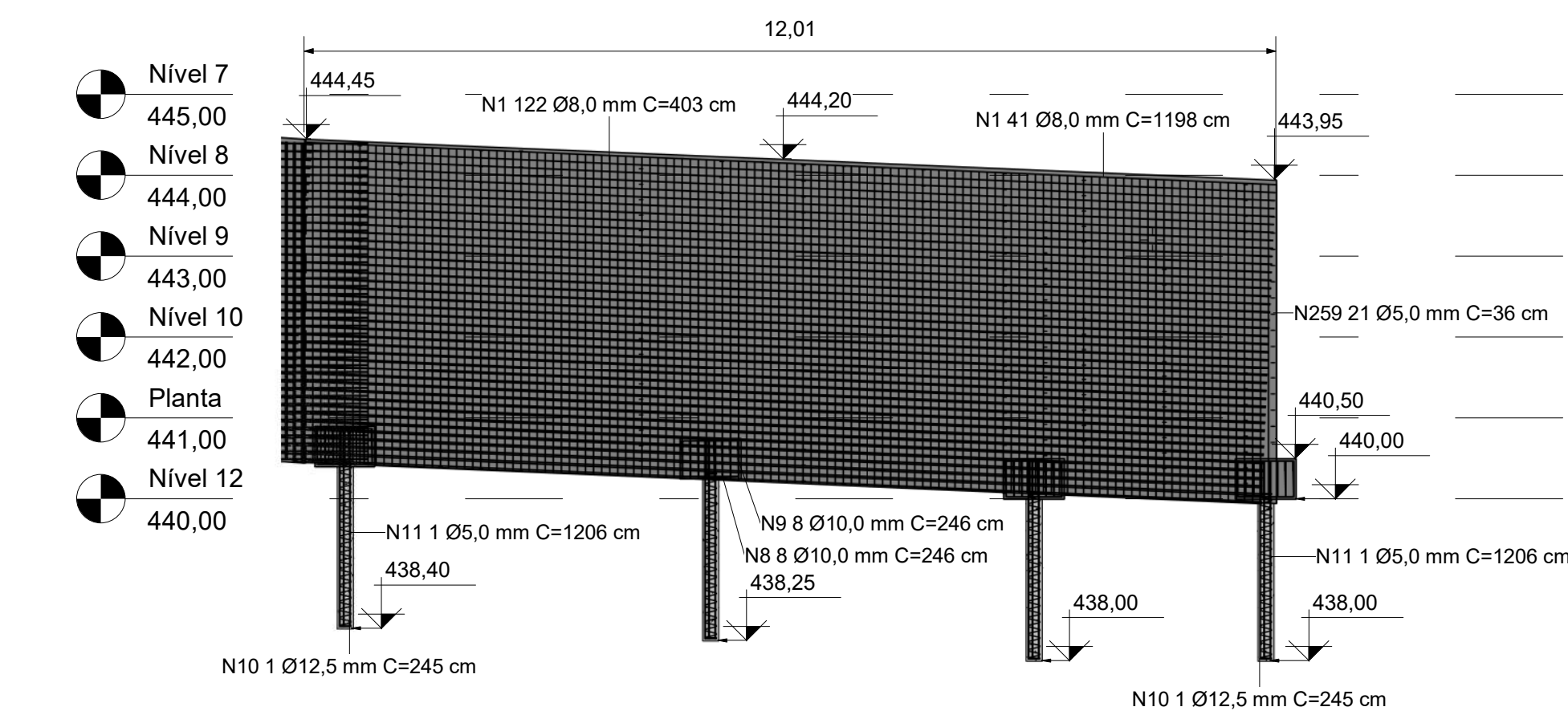
1 Seção 01 1 : 75
