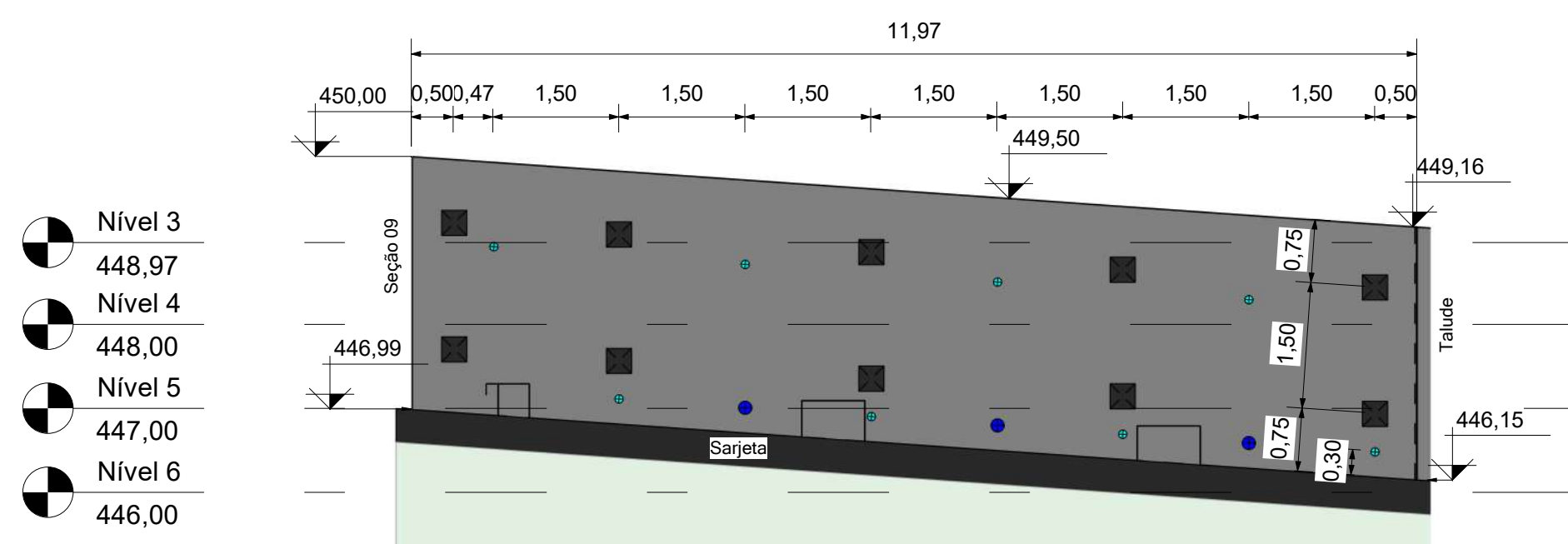
10 Seção 10 - Vista frontal 1 : 75
