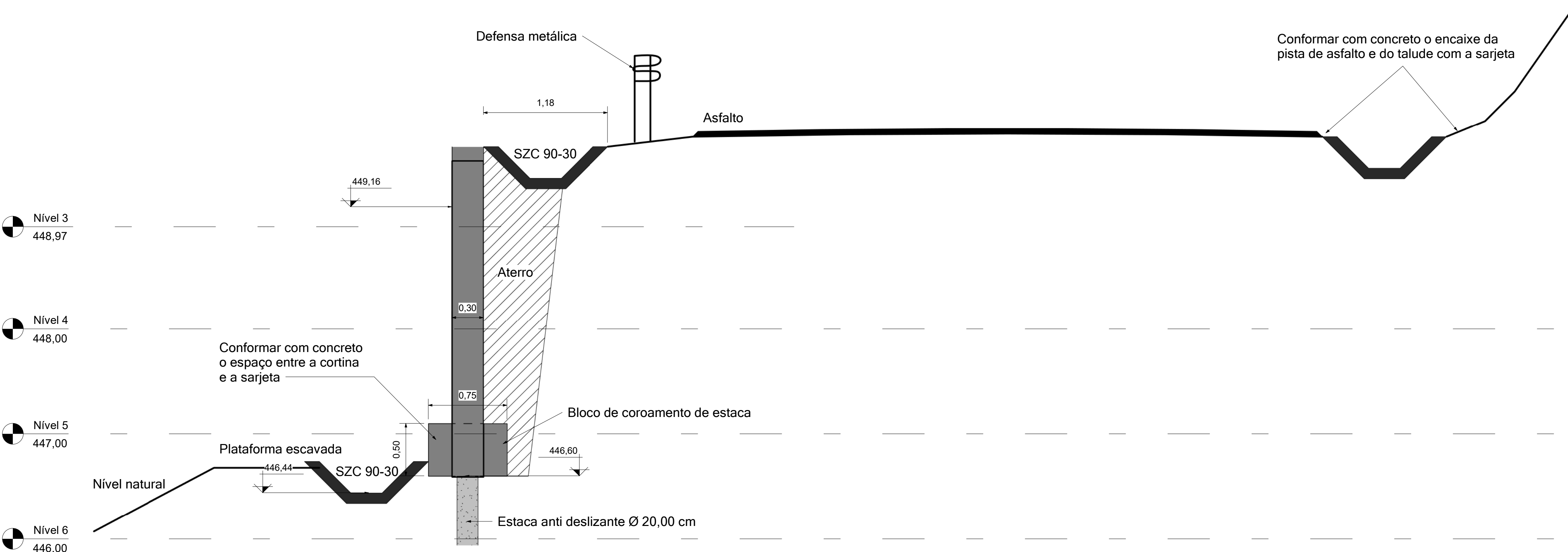
3 Corte de Drenagem Superficial 1 : 25
