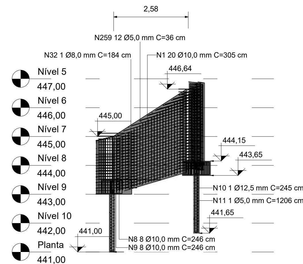
6 Seção 06 1 : 75
