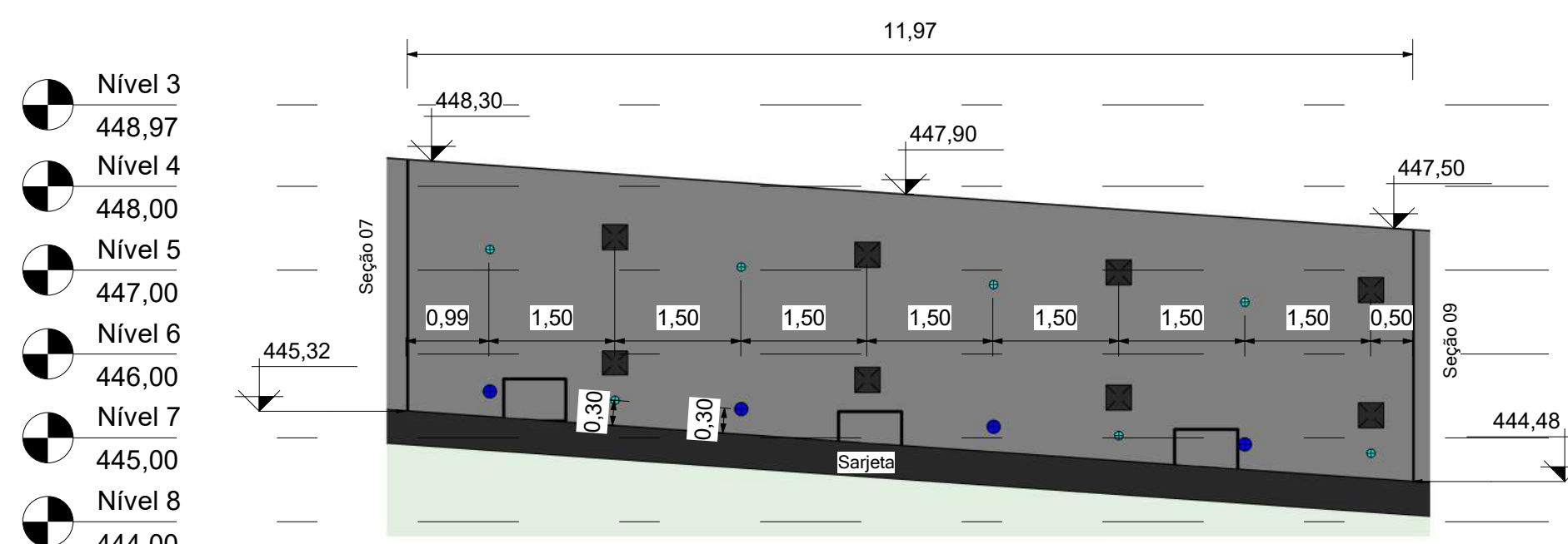
8 Seção 08 - Vista frontal 1 : 75
