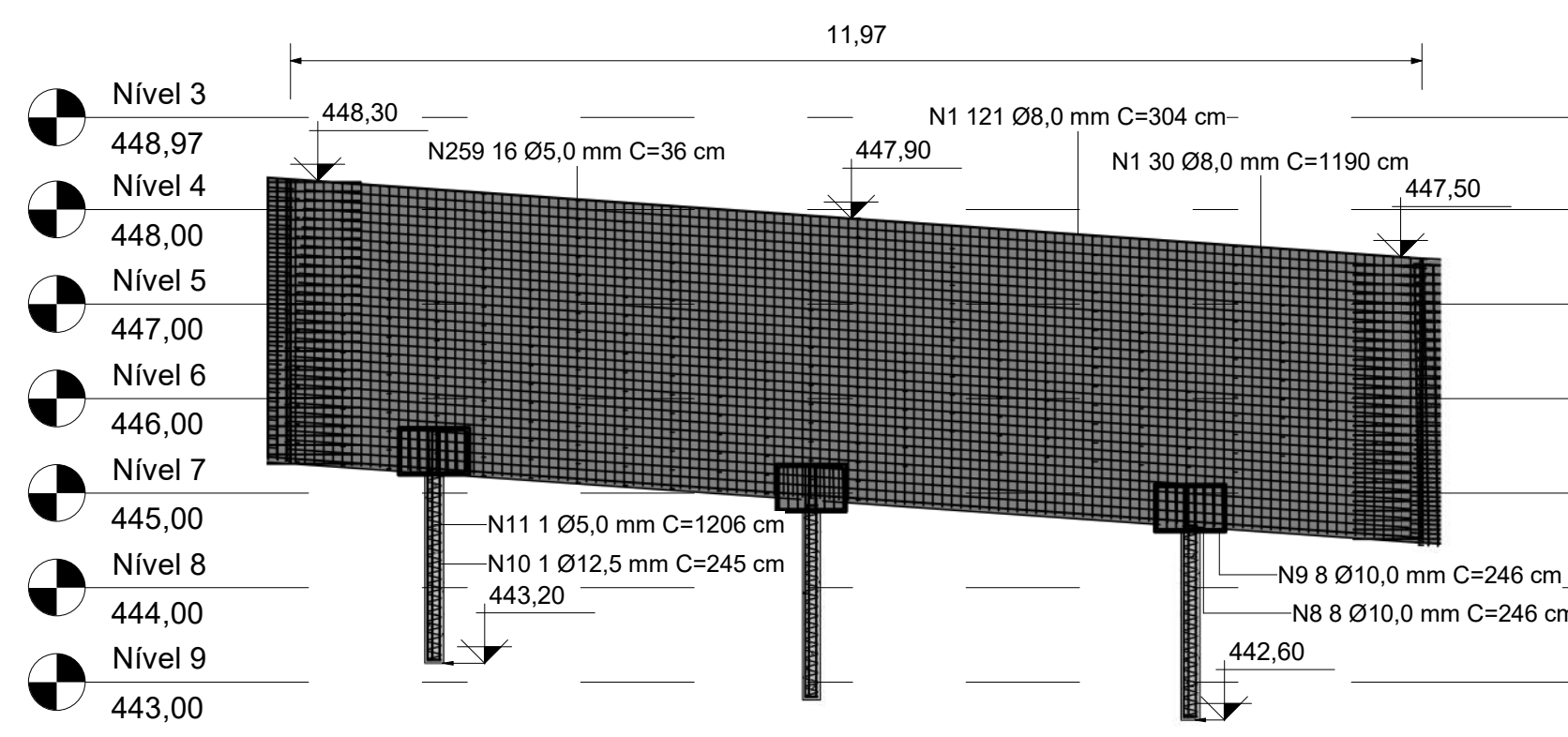
8 Seção 08 1 : 75
