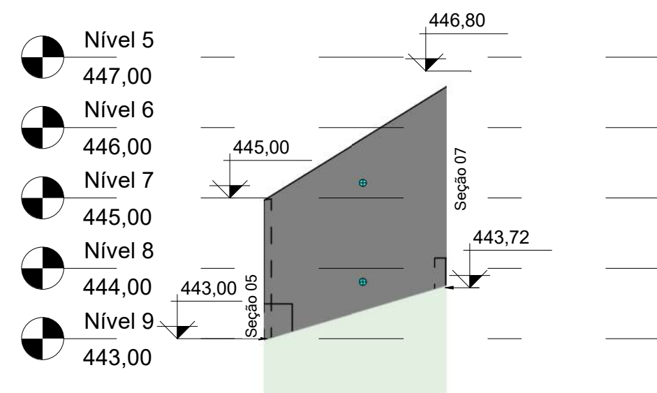
6 Seção 06 - Vista frontal 1 : 75
