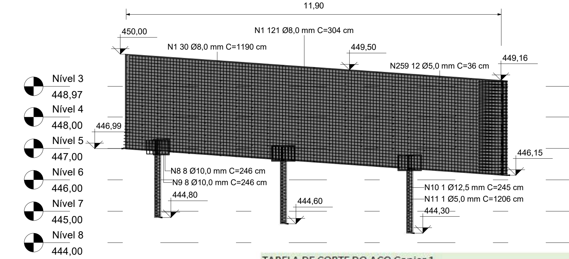
10 Seção 10 1 : 75
