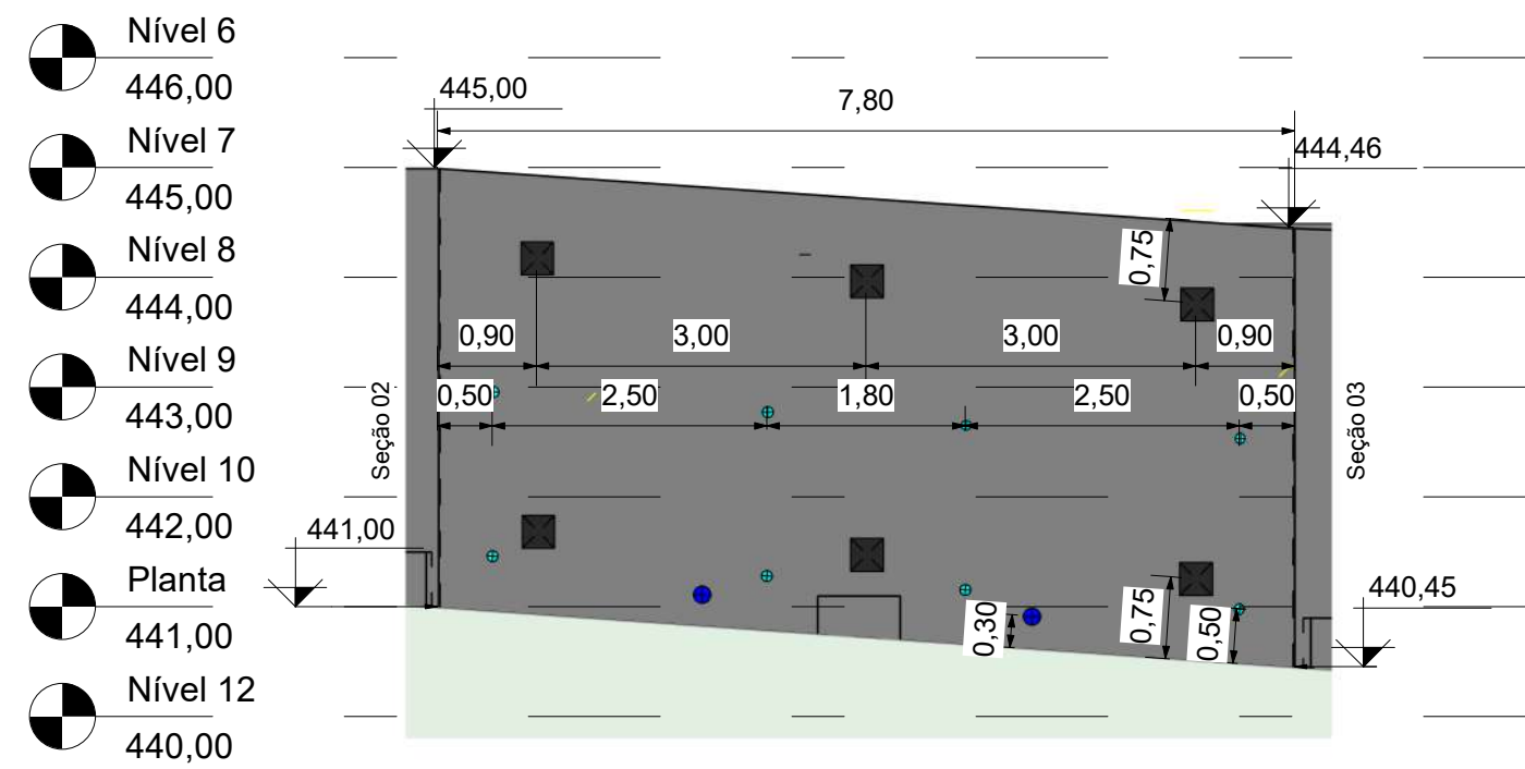
2 Seção 02 - Vista Frontal 1 : 75
