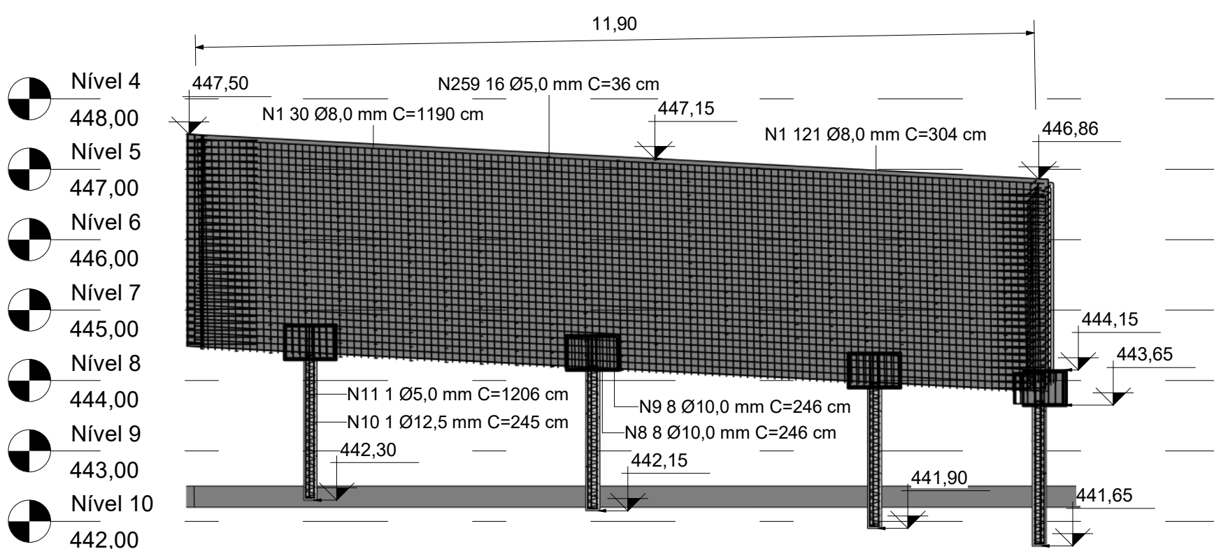
7 Seção 07 1 : 75
