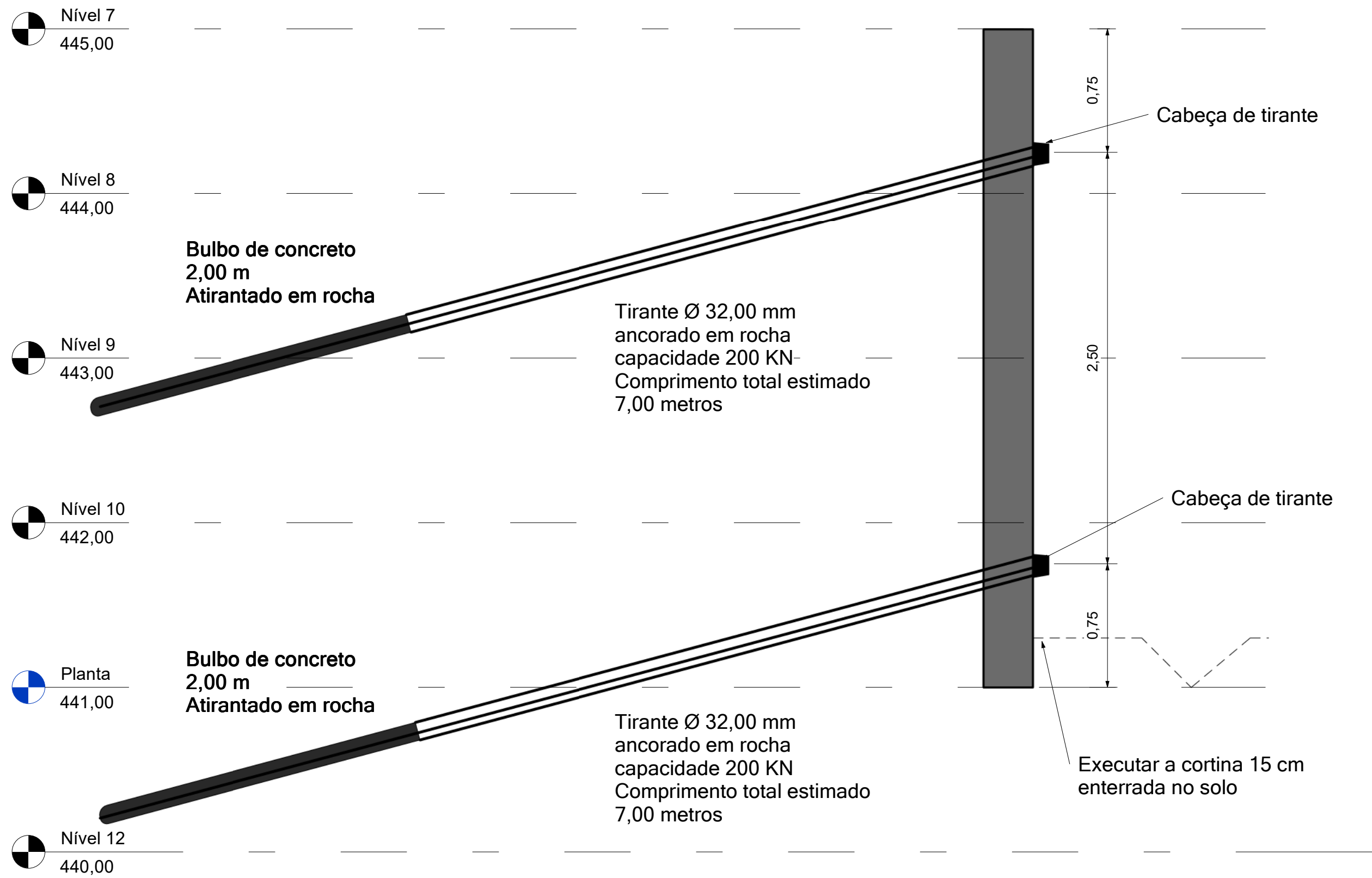
1 Tirantes 1 : 25
