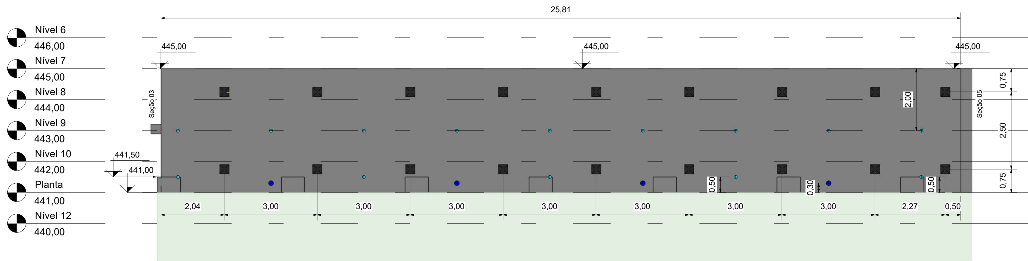
4 Seção 04 - Vista frontal 1 : 75
