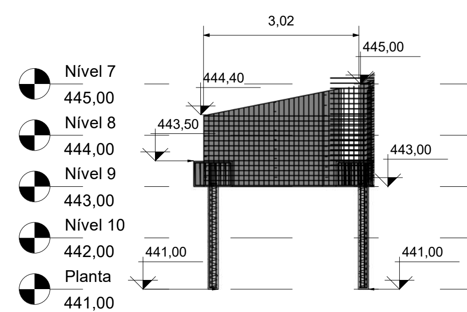
5 Seção 05 1 : 75
