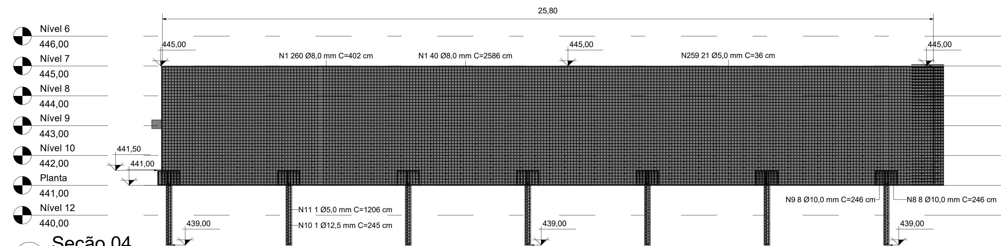
4 Seção 04 1 : 75
