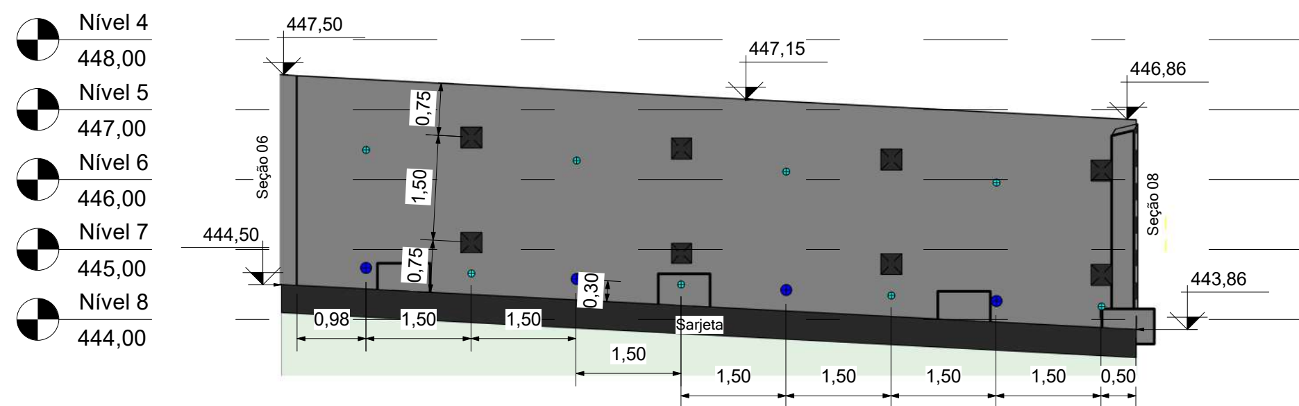
7 Seção 07 - Vista frontal 1 : 75
