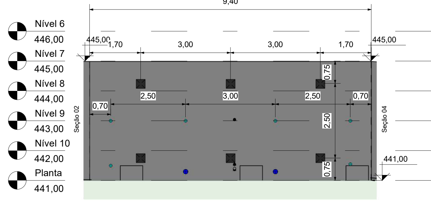
3 Seção 03 - Vista Frontal 1 : 75
