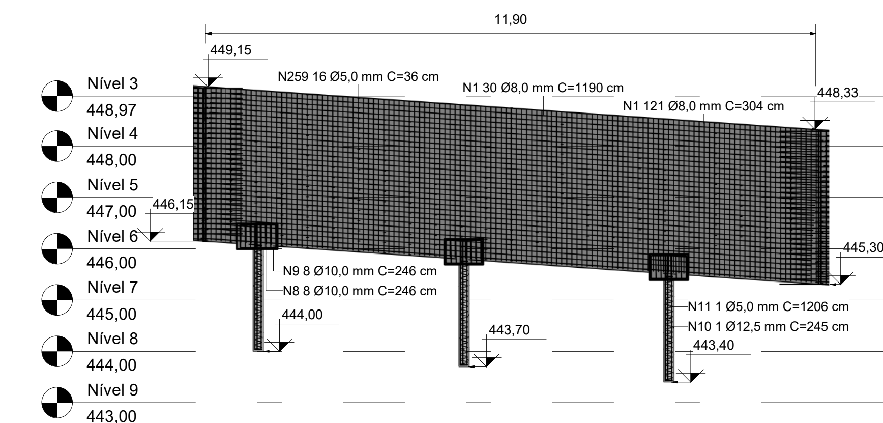
9 Seção 09 1 : 75
