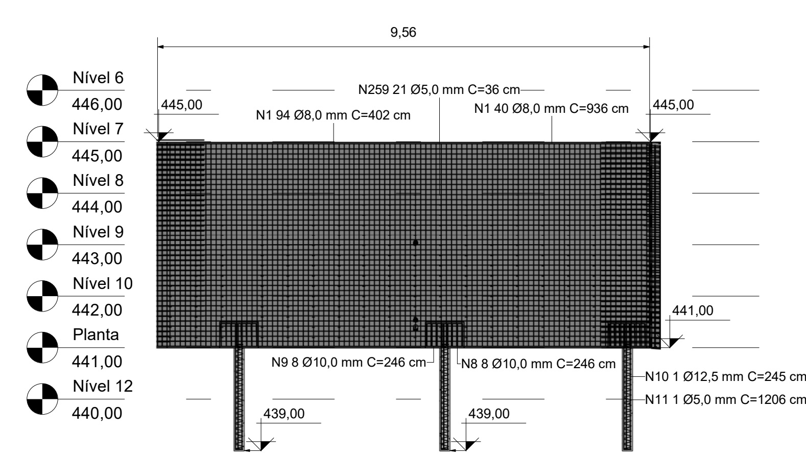
3 Seção 03 1 : 75
