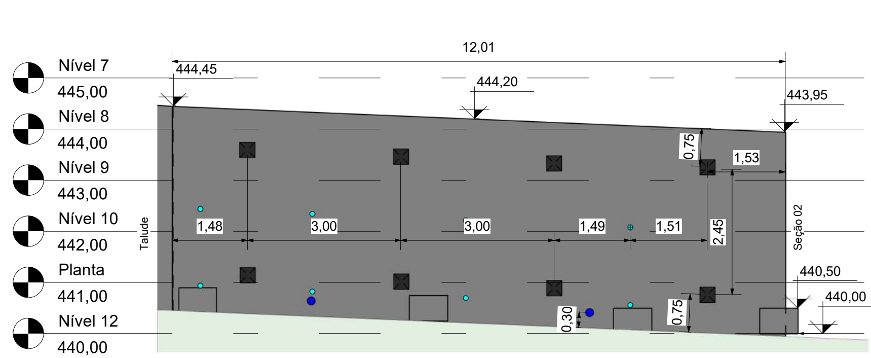
1 Seção 01 - Vista frontal 1 : 75
